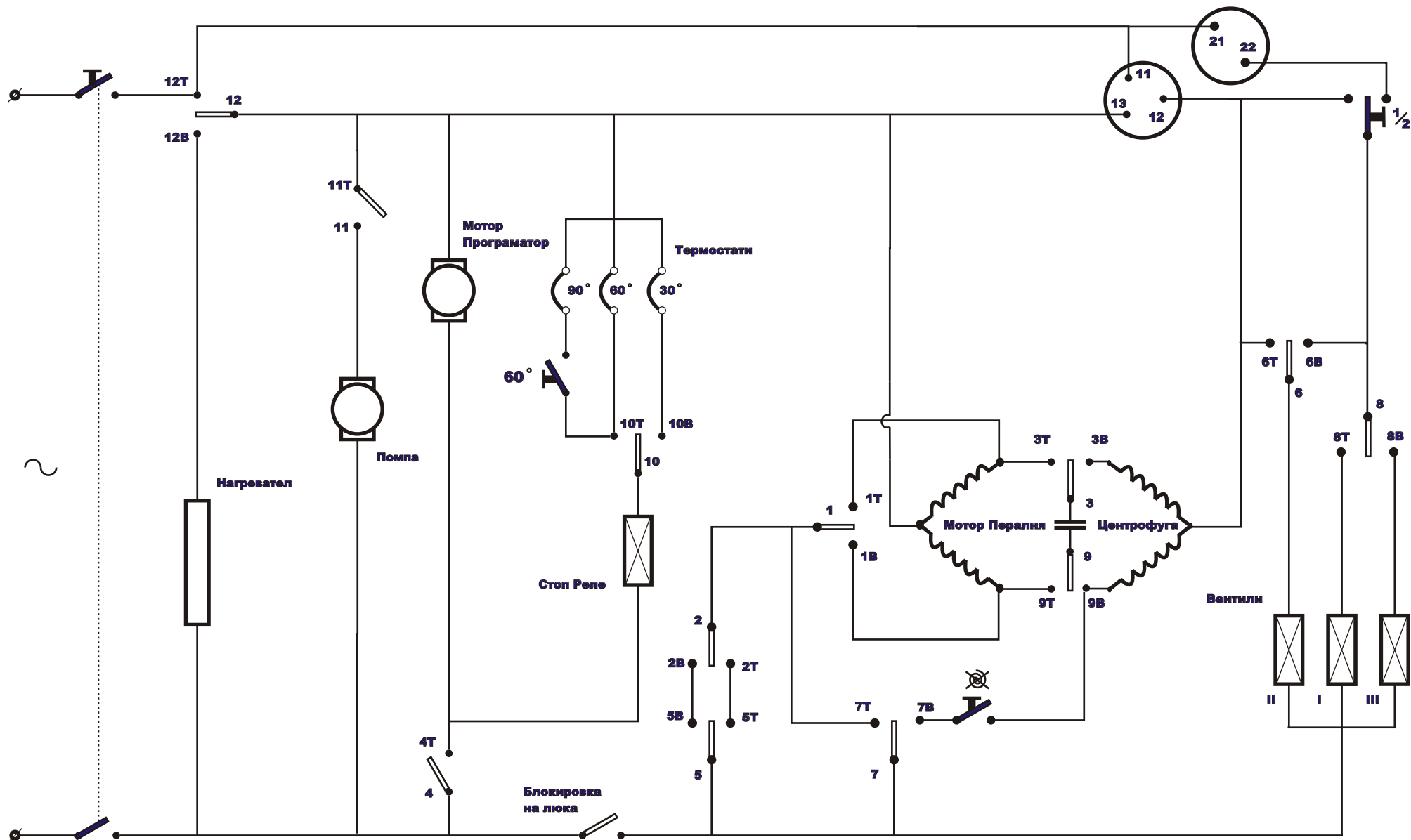
Принципна схема на "ПЕРЛА" 05 - програматор 900-01
